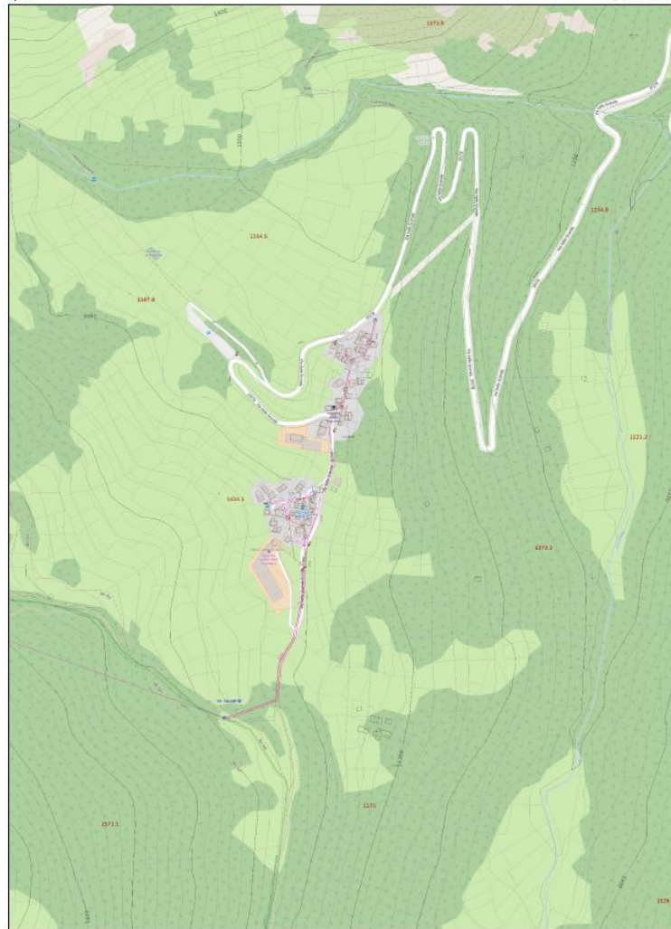
Figura 2 – Cartografia di rete in ambito extraurbano (scala 1:1.000) utilizzata per l'operazione c): diagnosi dell'anomalia di bassa pressione.
